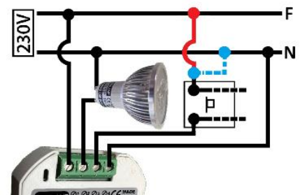
ESQUEMA DE CONEXIÓN
